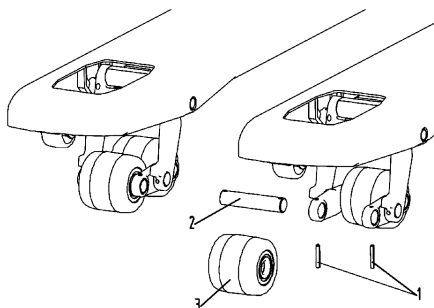
Fig. 10 – Roda dianteira
