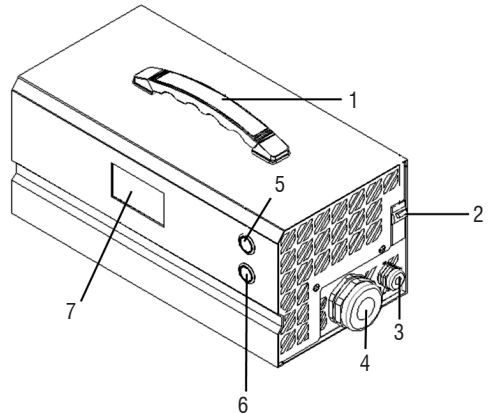
Fig. 6 – Componentes do carregador
