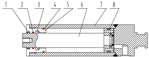
Fig. 9 – Estructura del cilindro de elevación
