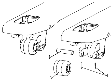
Fig. 10 – Rueda delantera
