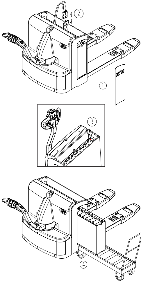
Fig. 8 – Substituição da bateria
