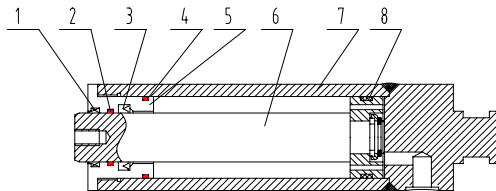
Fig. 9 – Estrutura do cilindro de elevação
