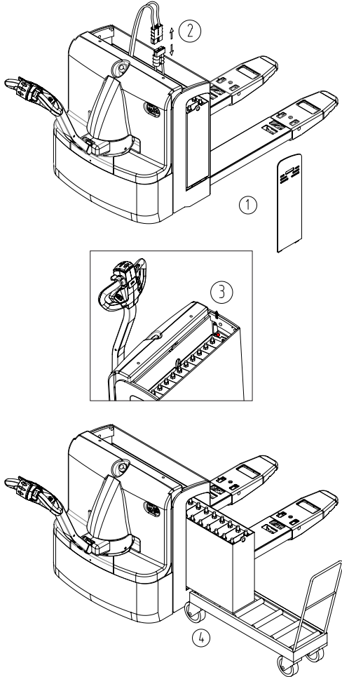
Fig. 8 – Sustitución de la batería
