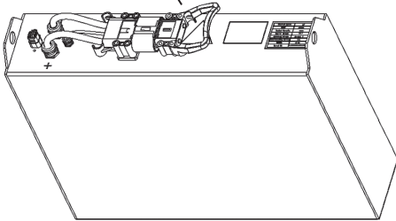
Fig. 5 – Plugue de alimentação
