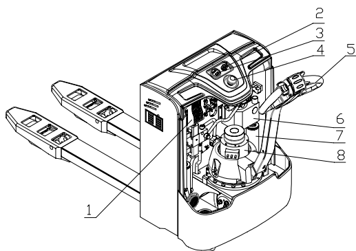
Fig. 1 – Componentes
